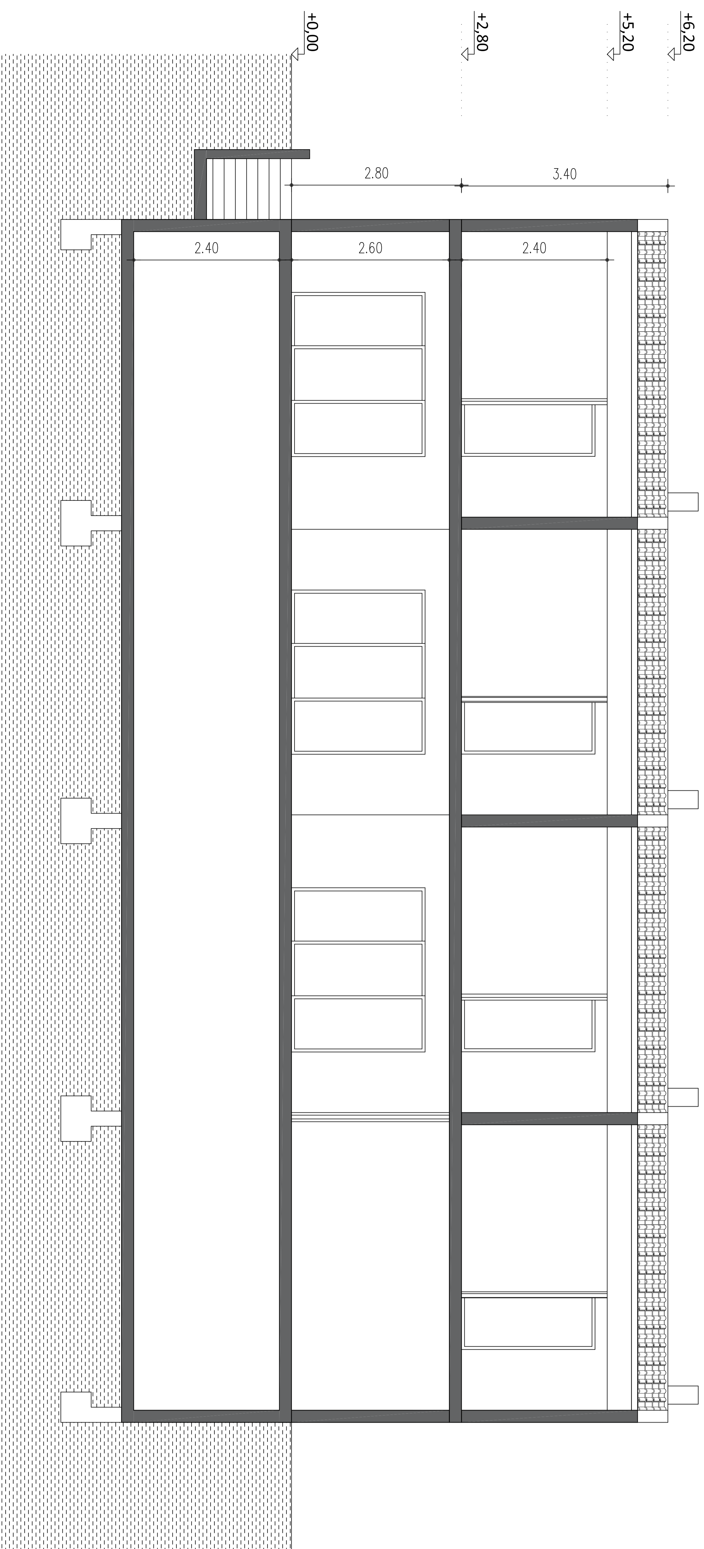
ΤΟΜΗ Α-Α' ΚΕΝΤΡΙΚΟΥ ΚΤΙΡΙΟΥ
